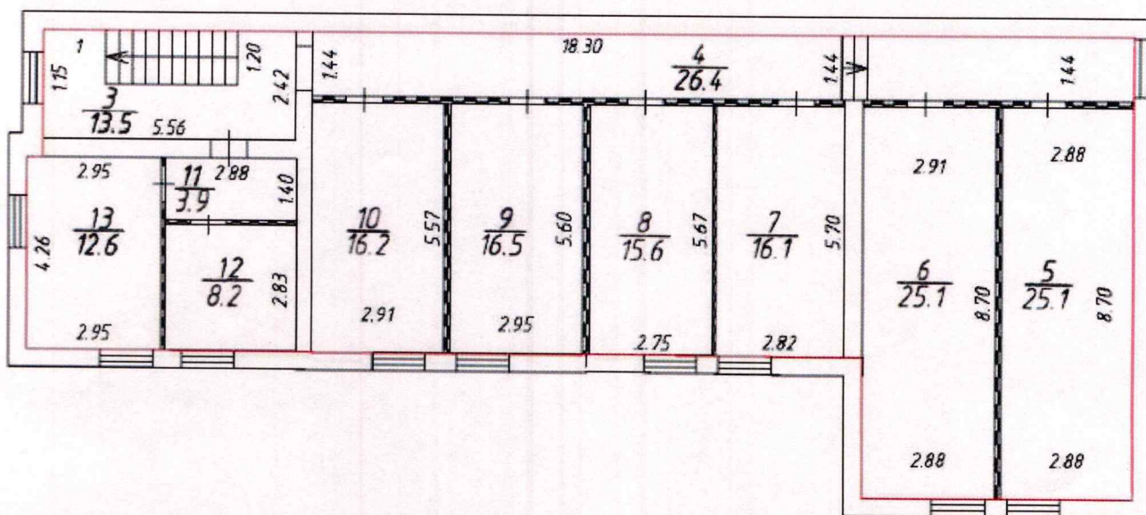
Этаж 2
